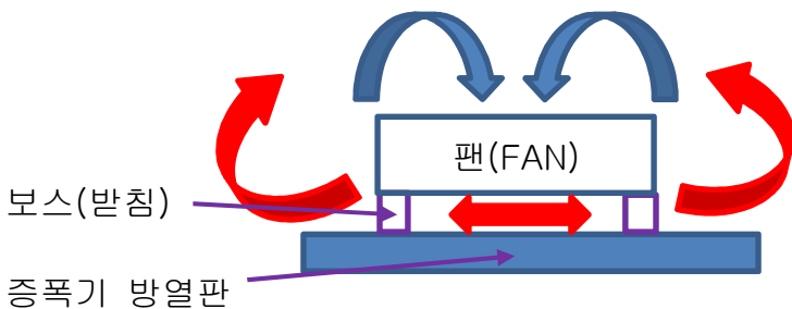
(별매의 PN-FAN-G6005 팬(FAN) 장착모양)
